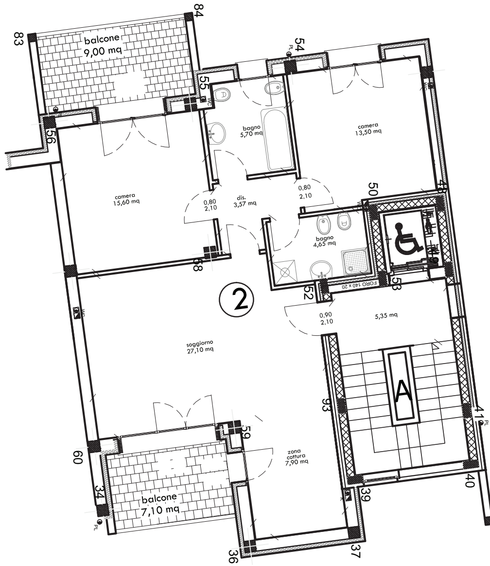
APPARTAMENTO A2 STATO DI PROGETTO
