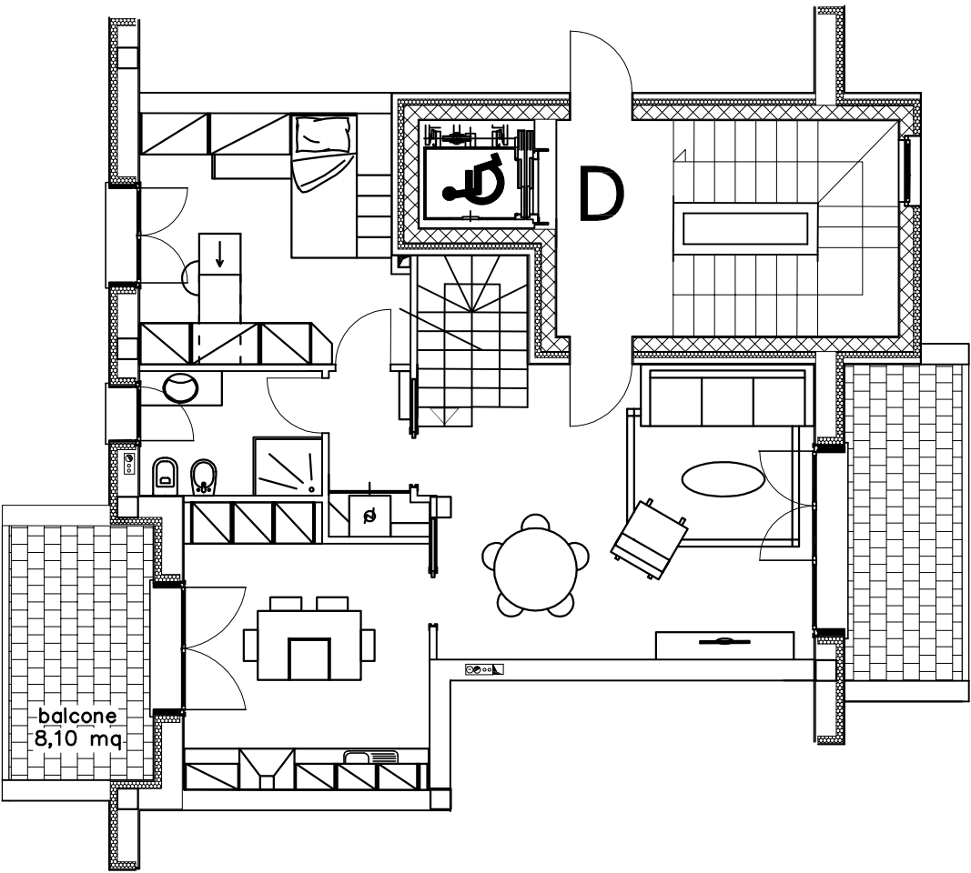
Appartamento D8 + Sottotetto
