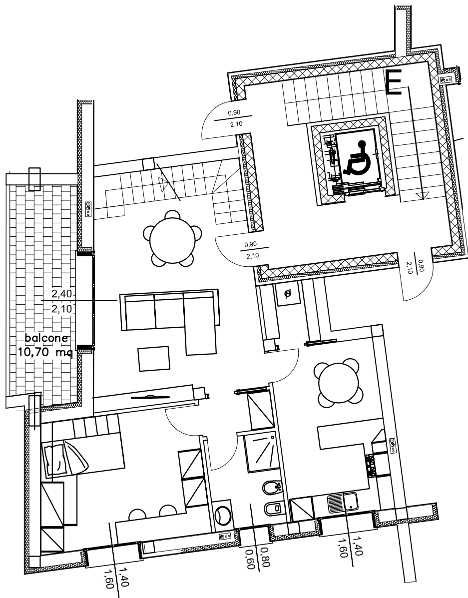
Appartamento E9 + Sottotetto
